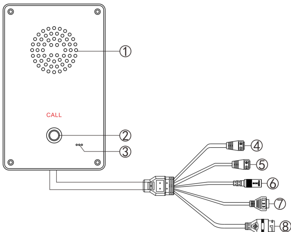
Рис. 2. Описание устройства
