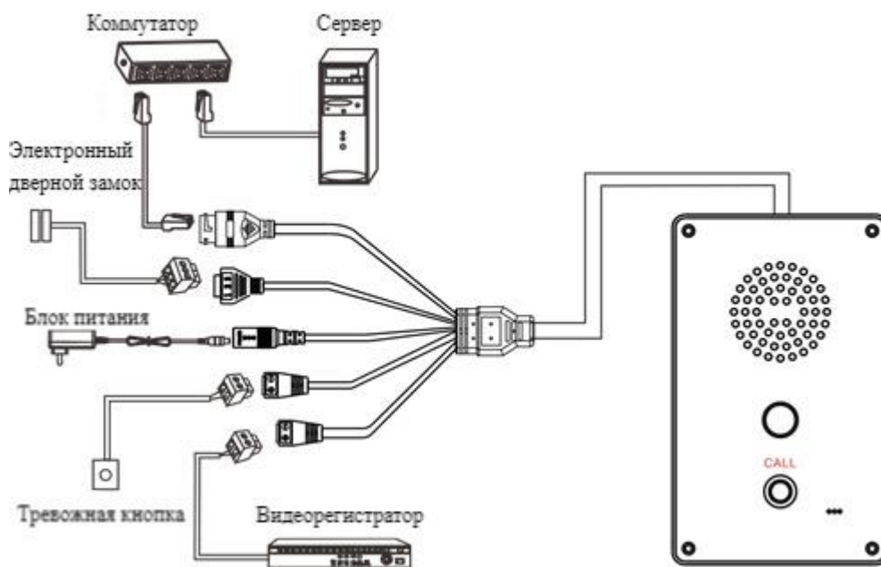
Рис. 4. Описание устройства
